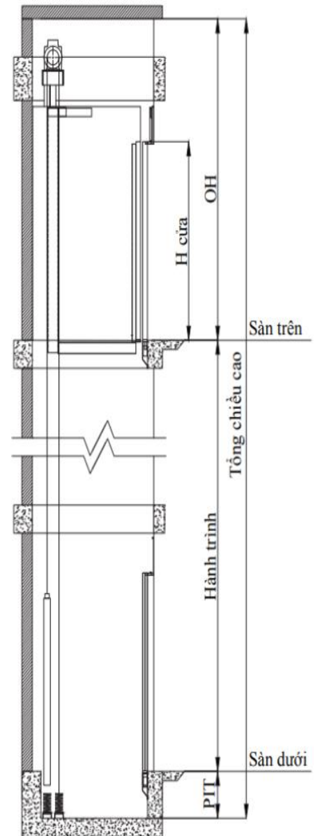
MẶT CẮT DỌC HỖ THANG
